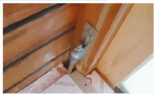
耐震金物の取付
